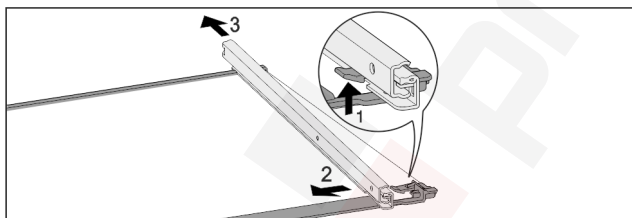
Fig. 84 Üveglap sínekkal
