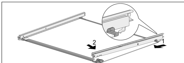
Fig. 85 Üveglap sínekkal
